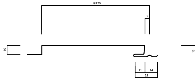
SSスパン F-120 一般断面図 1/1
