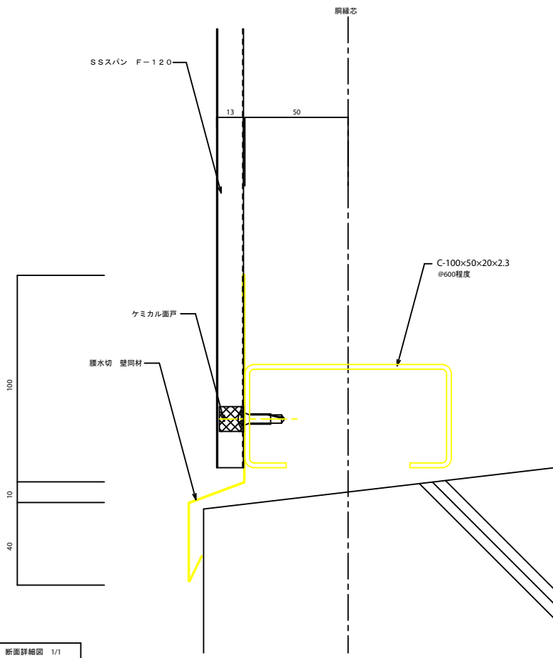
止水切 断面詳細図 1/1
